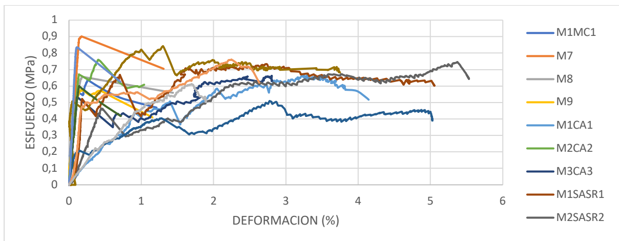
Figura 21: Gráfico esfuerzo – deformación de los elementos ensayados.
